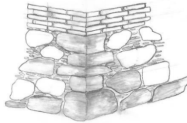
Γωνιακή λεπτομέρεια
