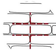
Σταυρωτό χτίσιμο
