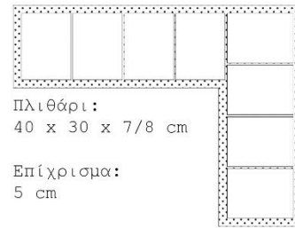
Γωνιακή λεπτομέρεια
